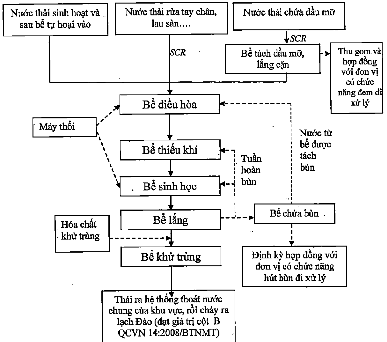
Sơ đồ hệ thống xử lý nước thải của dự án
